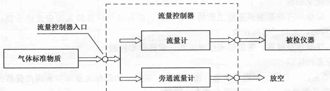
图 1 流量控制器
